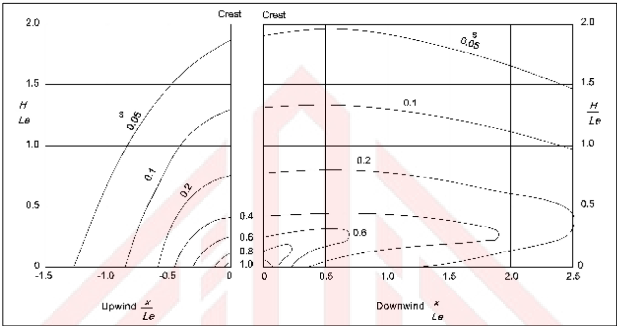
الشكل أ-2/1: المعامل الطبوغرافي (s) للأجراف والخنائق.
